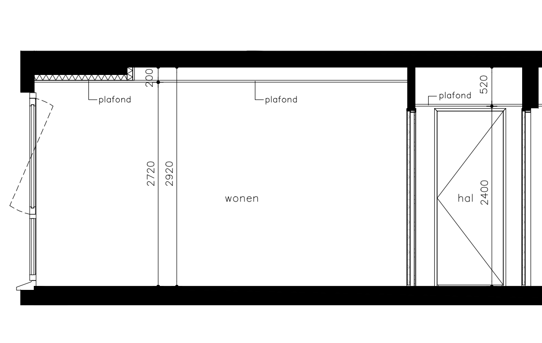
Doorsnede
